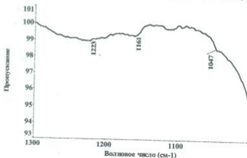
Рис. 10. ИК-спектр жидкой фазы в системе ZnS-унитиол-вода после автоматической коррекции базовой линии в диапазоне 1300\text{--}1000\text{ см}^{-1}
