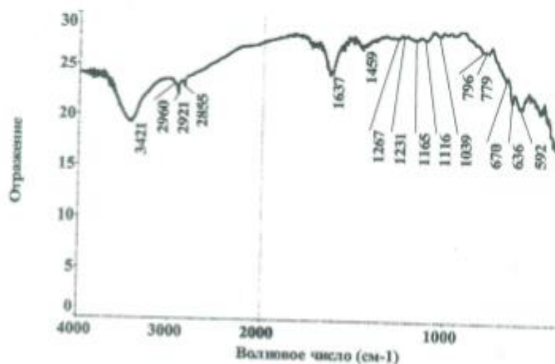
Рис. 11. ИК-спектр твердого остатка в системе ZnS-унитиол-вода
